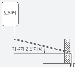
<하수구 또는 하천 등 외부로 직접 배수할 경우>
