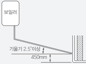
<실내의 배수구로 배수할 경우>
