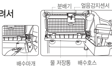
배수마개
