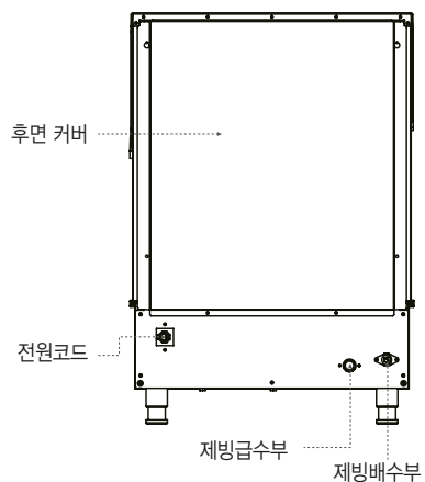
■ 후면도
