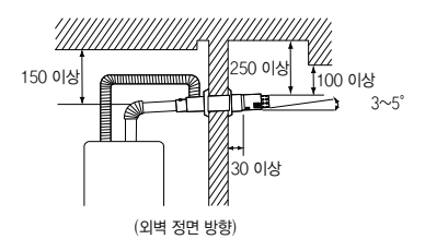
[벽면과 이격거리 제한] (단위:mm)
