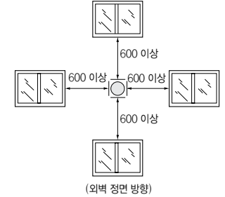
[터미널(배기통)에서 창문까지의 거리 제한] (단위:mm)
