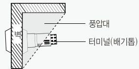
풍압대 : 바람이 불 때 건물벽의 영향으로 대기압 보다 기압이 높아지는 지역
