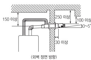
[벽면과 이격거리 제한] (단위:mm)
