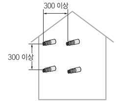
[급배기통을 여러개 설치할 경우의 거리 제한] (단위:mm)
